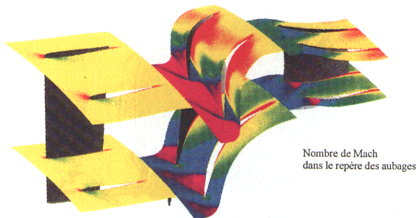
Fig 6 : Calcul NS3D sur le 1 er étage complet d'un compresseur HP. Sections proches du moyeu et du carter
