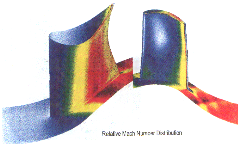
Fig 10 : Calcul NS3D sur la turbine HP du M88-2 Distribution du nombre de Mach relatif près des parois des aubes
