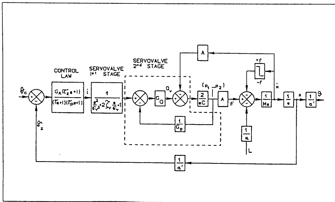
Fig. 10 - VACU Servoloop Block Diagram
