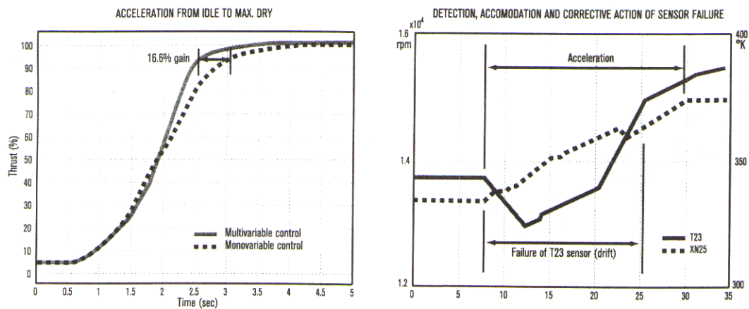
Fig 5 : Illustration des avantages des techniques de régulation multi-variables : temps d'accélération réduit, atténuation des effets de pannes
