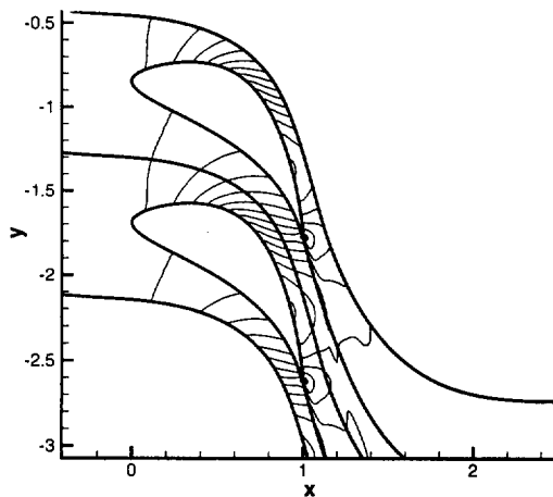
Fig. 16 : Blade geometry : nozzle blade
