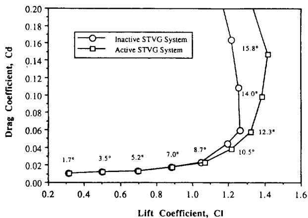
b) NACA 4415 drag polar
