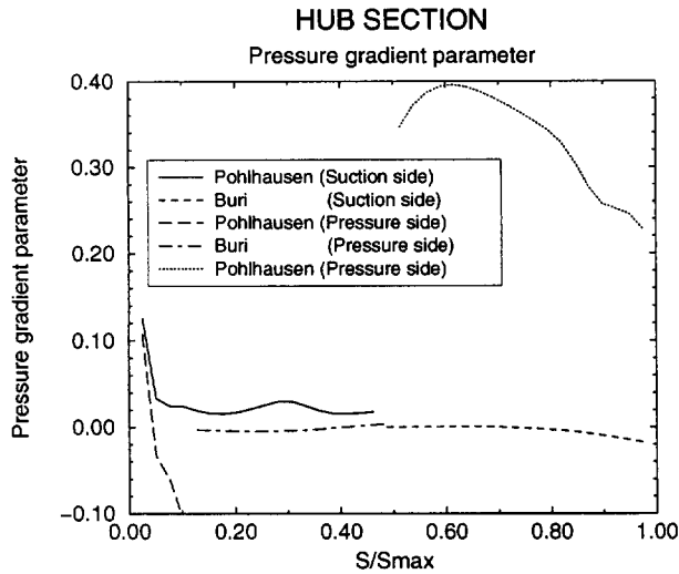
Fig. 15 : Pressure gradient parameter
