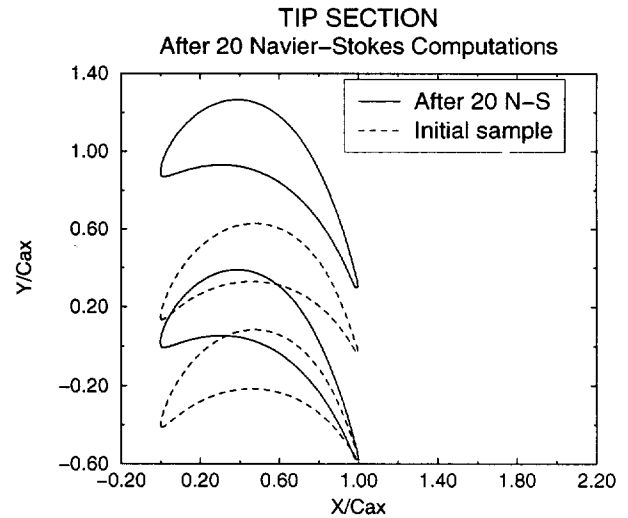
Fig. 7 : Blade geometries : tip section
