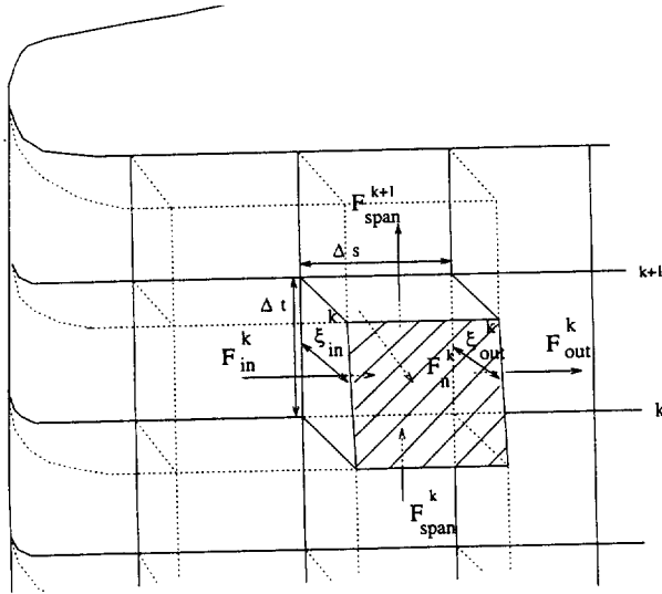
Fig. 2 : 3D transpiration
