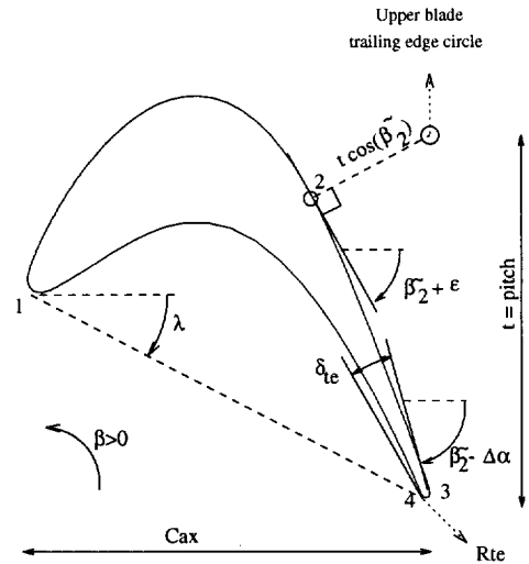
Fig. 2 : Geometry model : basic parameters
